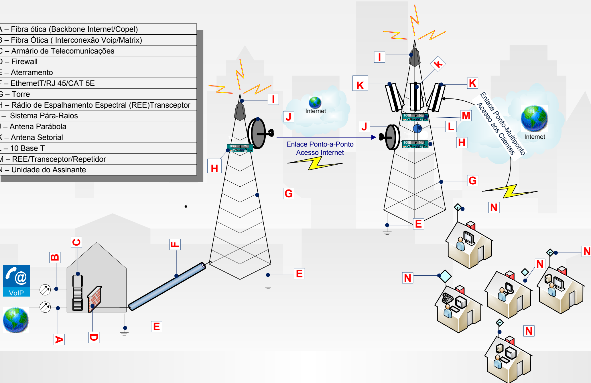
Diagrama 02 - Rede Sem Fio
