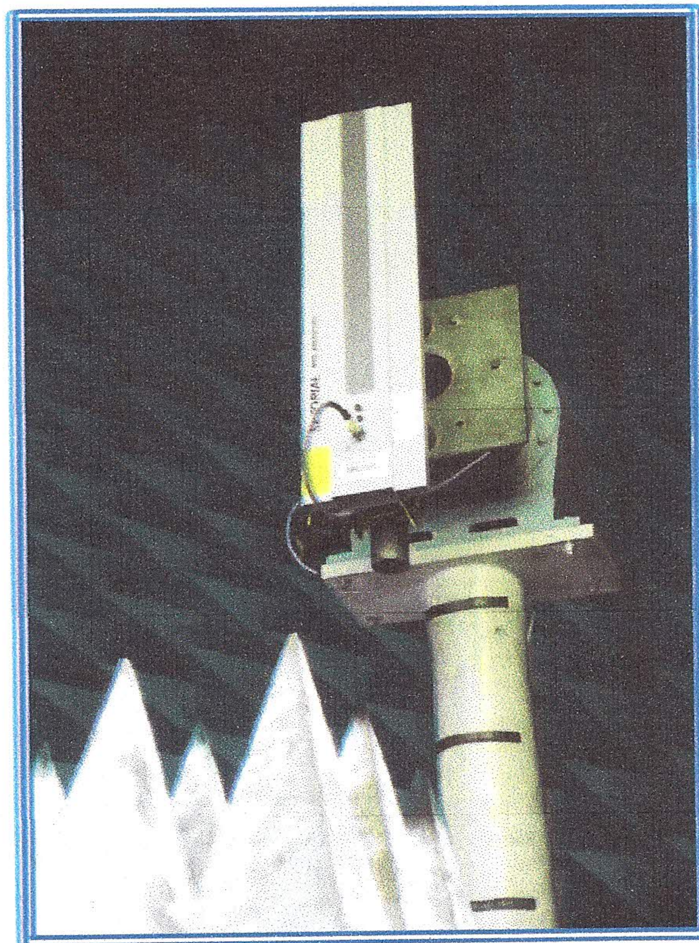
Figura 1 – Antena sob teste.
