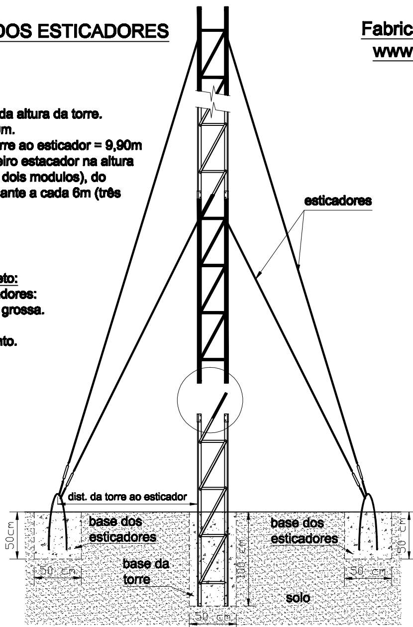
VISTA LATERAL
