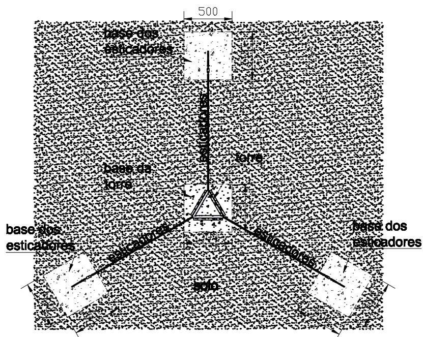
VISTA SUPERIOR
