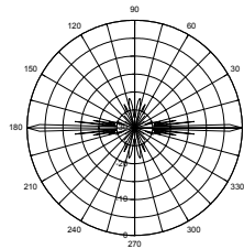
Omni 15 dBi
